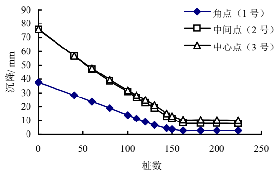
图1 沉降与桩数关系曲线
