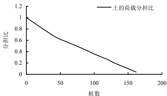
图2 土的荷载分担比与桩数关系曲线
